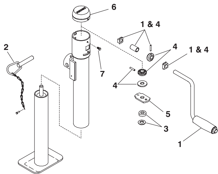
Hitchjack - Fulton
